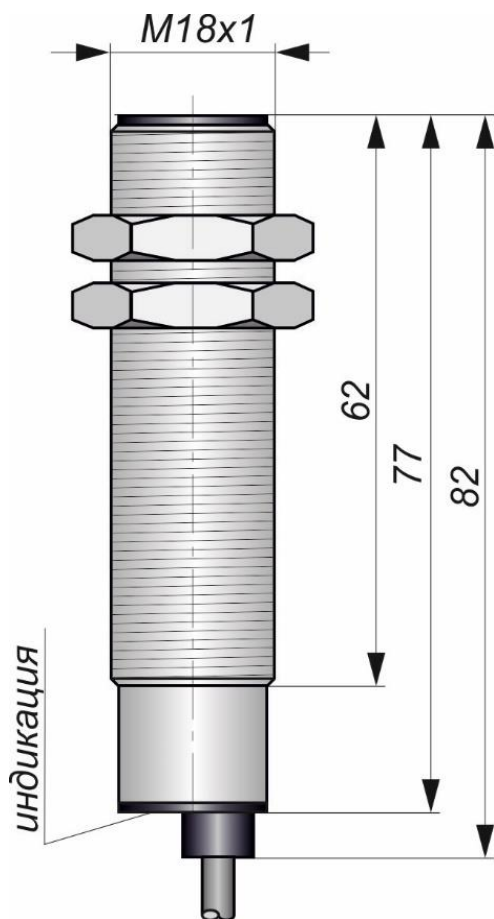
Габаритный чертеж
