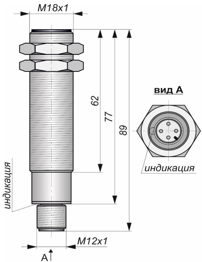
Габаритный чертеж
