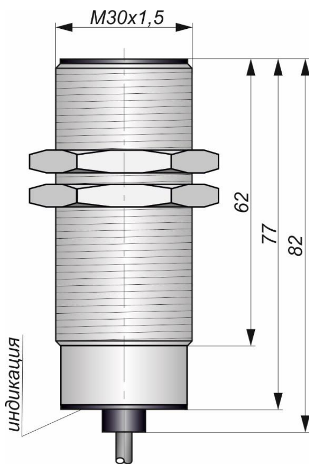
Габаритный чертеж
