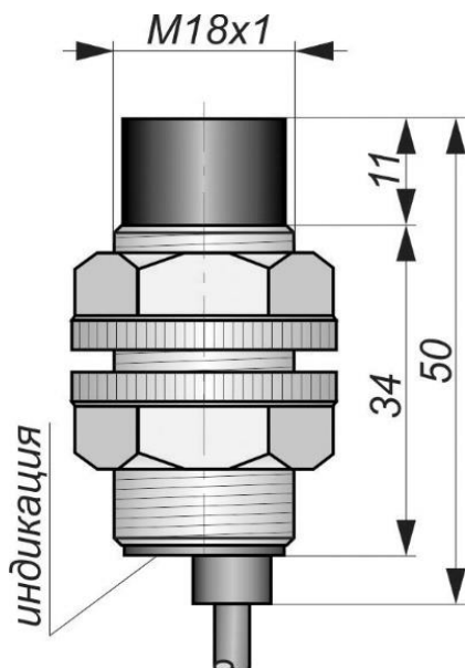
Габаритный чертеж
