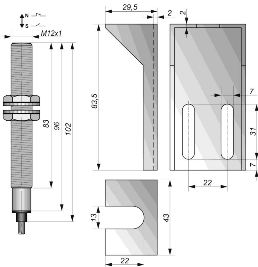
Габаритный чертеж
