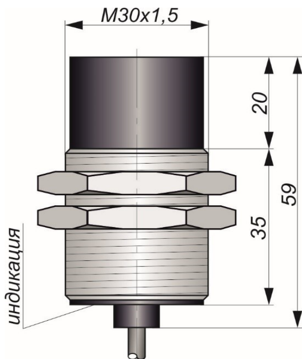
Габаритный чертеж
