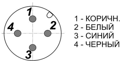
Цоколевка разъема
