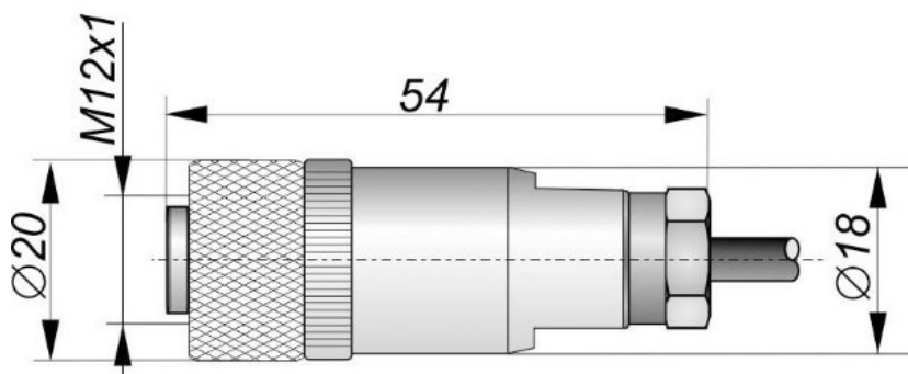
Габаритный чертеж
