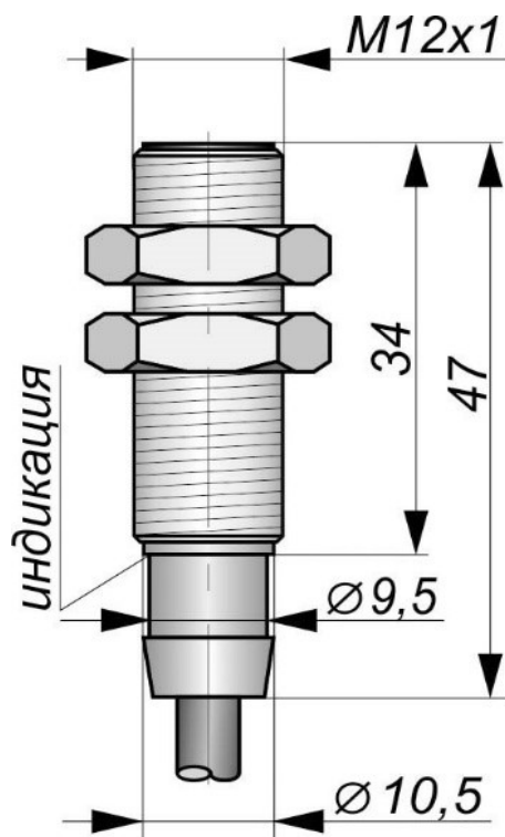
Габаритный чертеж
