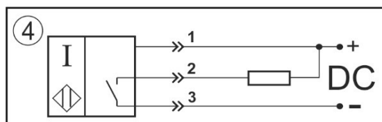
Нормально-разомкнутый контакт
