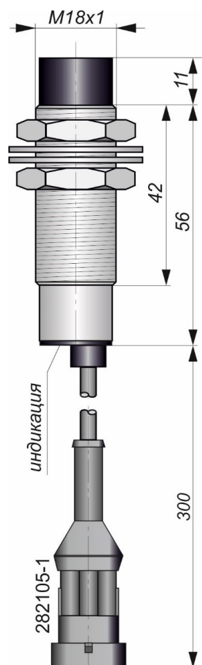
Габаритный чертеж
