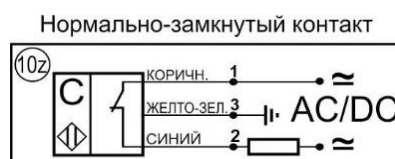
Схема соединения
