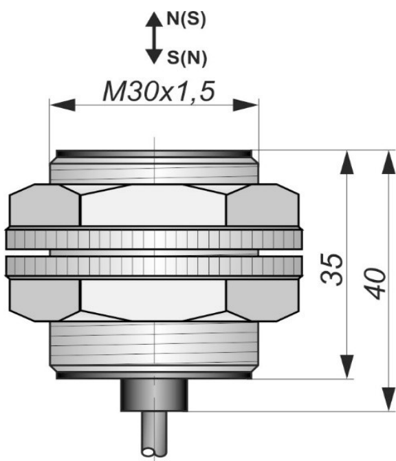
Габаритный чертеж
