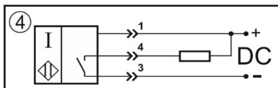
Цоколевка разъема
