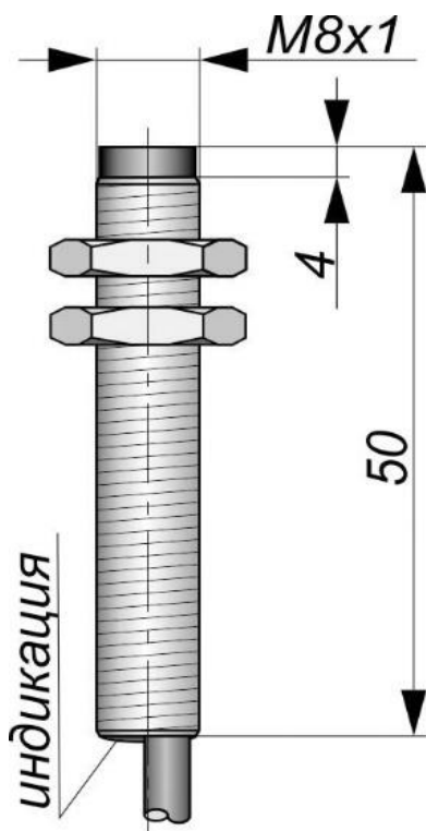
Габаритный чертеж
