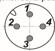
Цоколевка разъема
