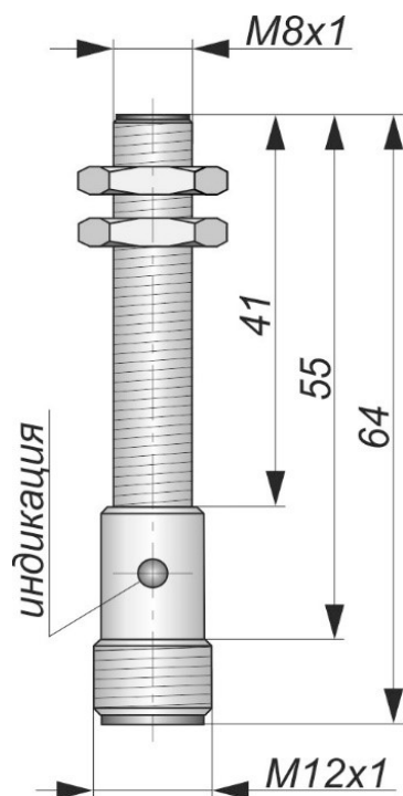
Габаритный чертеж
