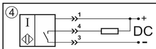
Цоколевка разъема
