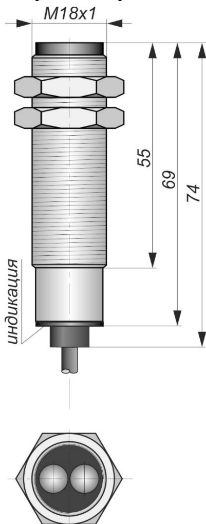
Габаритный чертеж
