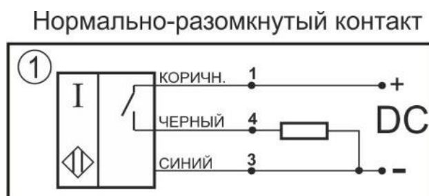
Схема соединения
