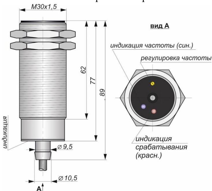
Габаритный чертеж
