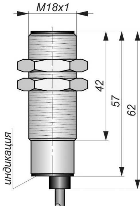
Габаритный чертеж
