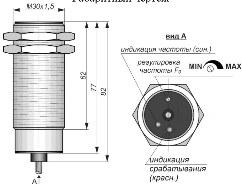
Габаритный чертеж
