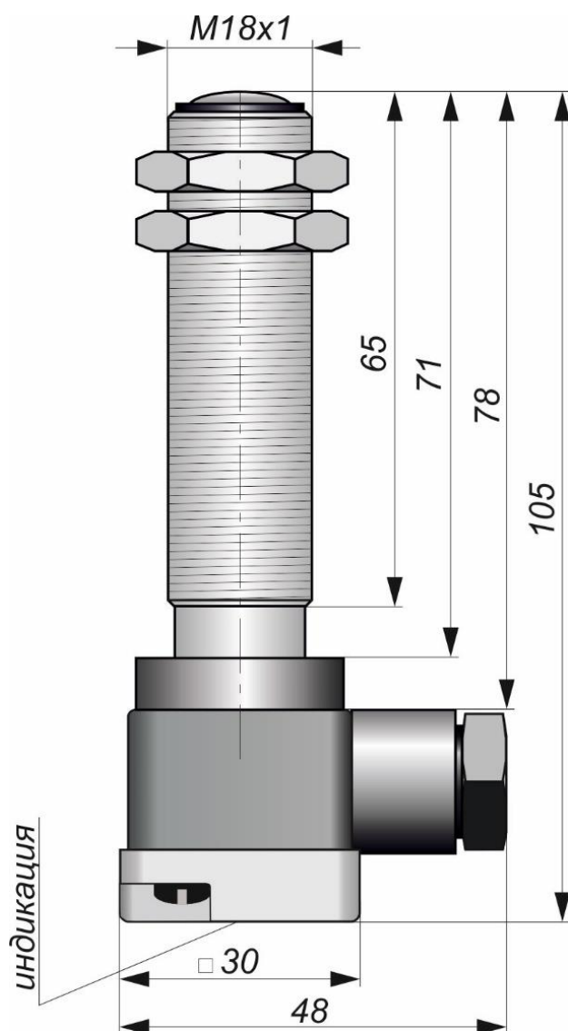
Габаритный чертеж
