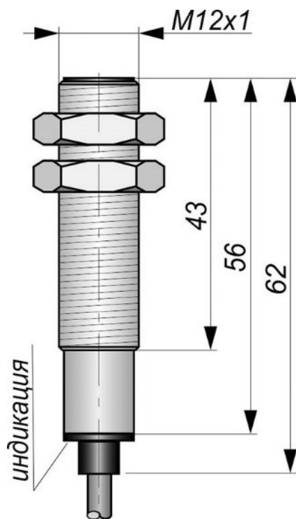
Габаритный чертеж
