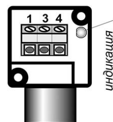
Цолевка клеммной колодки
