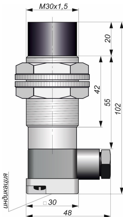
Габаритный чертеж
