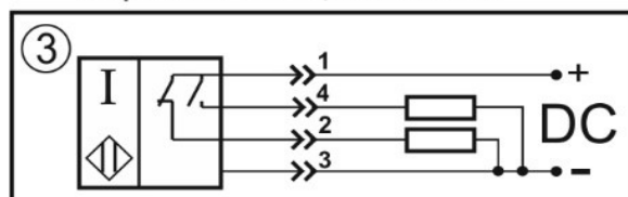
Переключающий контакт
