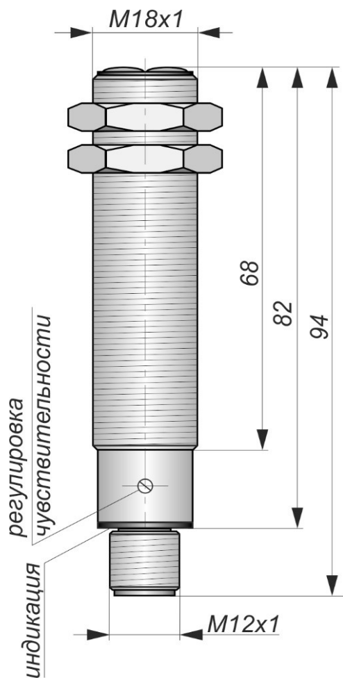
Габаритный чертеж
