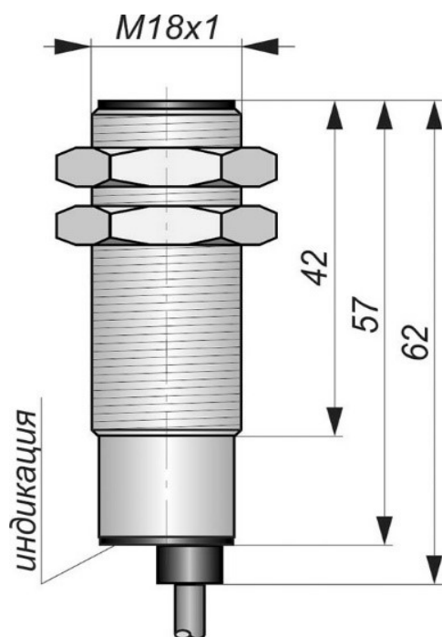
Габаритный чертеж
