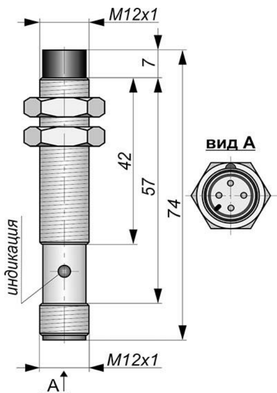
Габаритный чертеж
