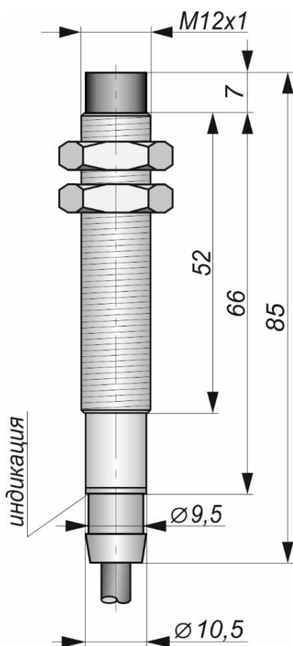
Габаритный чертеж
