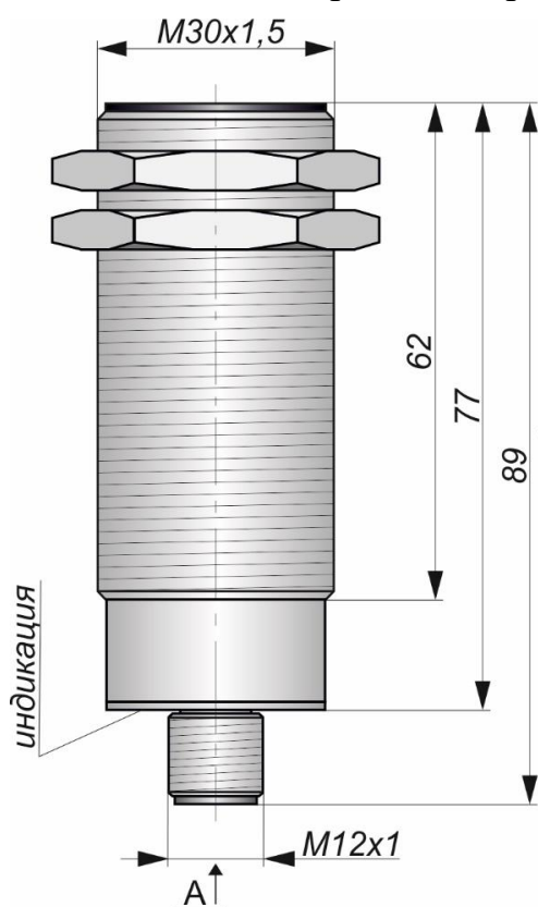
Габаритный чертеж
