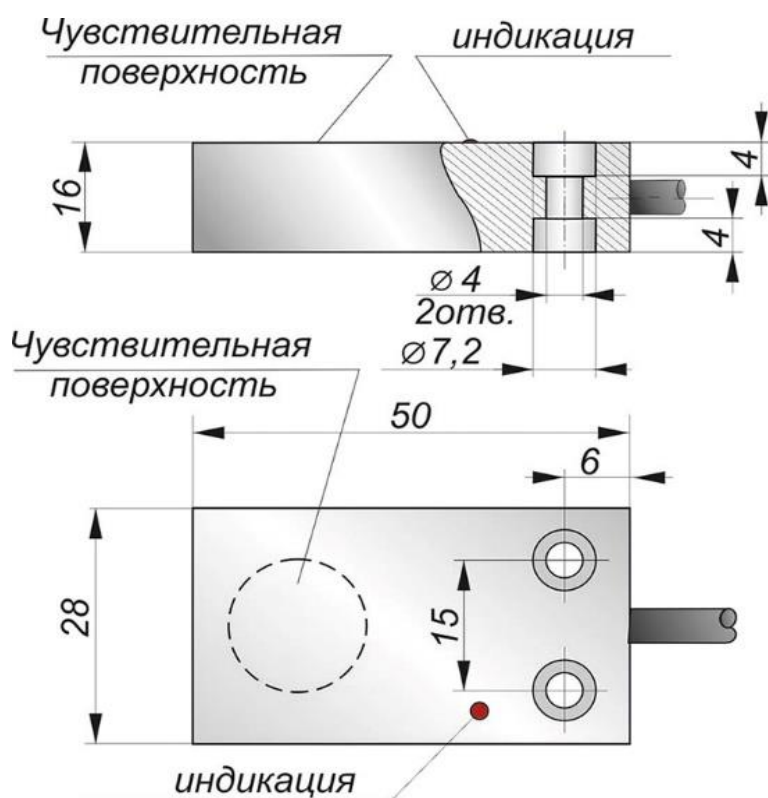
Габаритный чертеж
