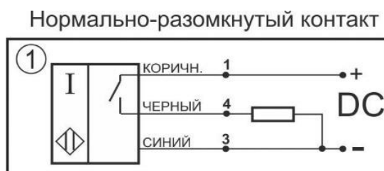
Схема соединения
