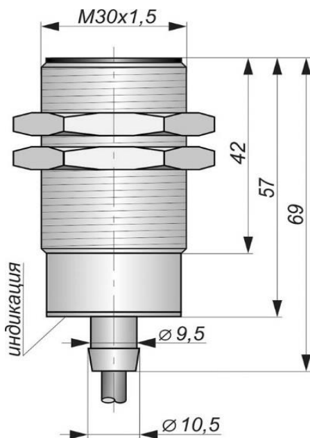
Габаритный чертеж
