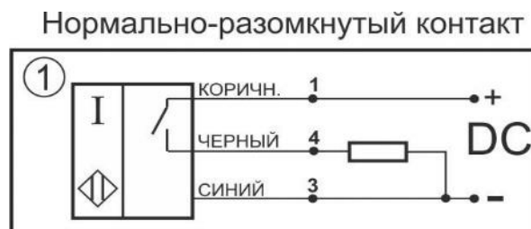
Схема соединения
