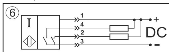
Переключающий контакт
