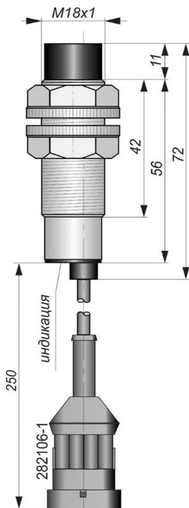
Габаритный чертеж
