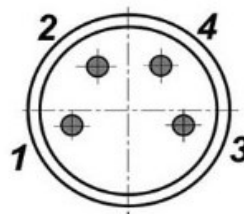
Цоколевка разъема
