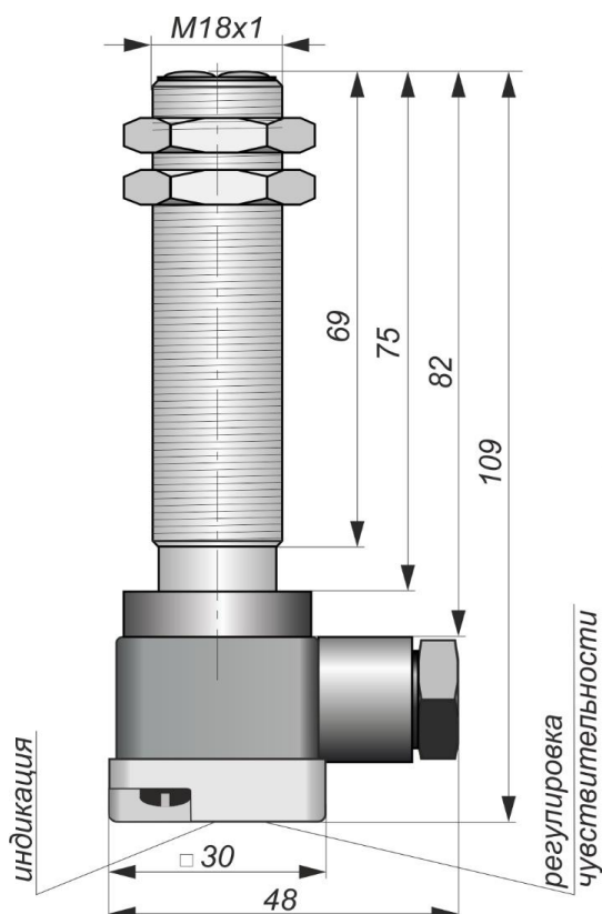
Габаритный чертеж
