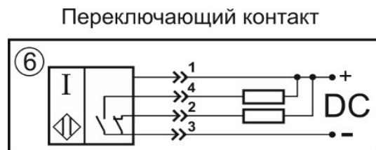
Схема соединения
