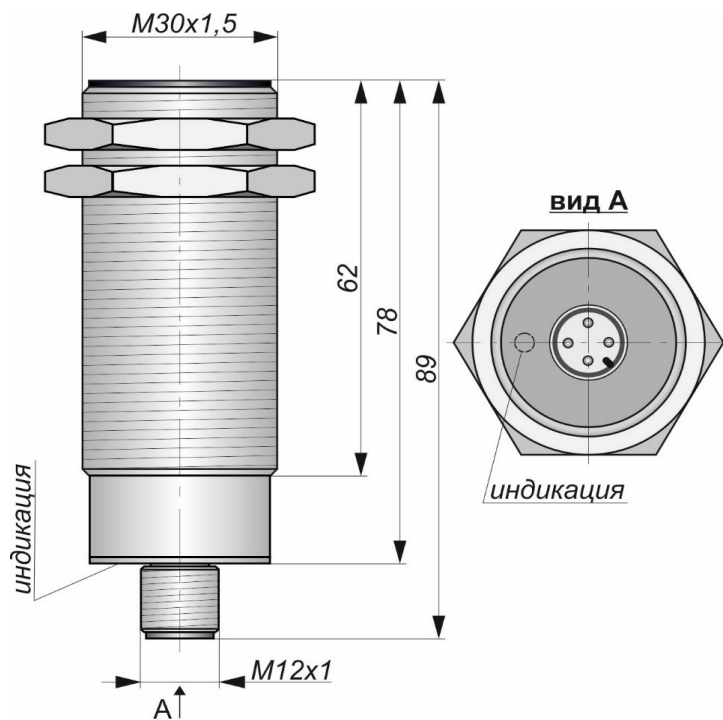
Габаритный чертеж
