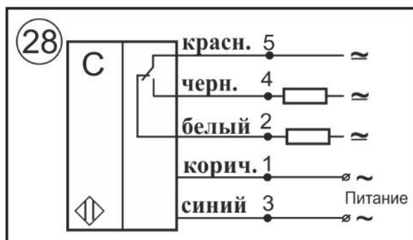
Схема соединения
