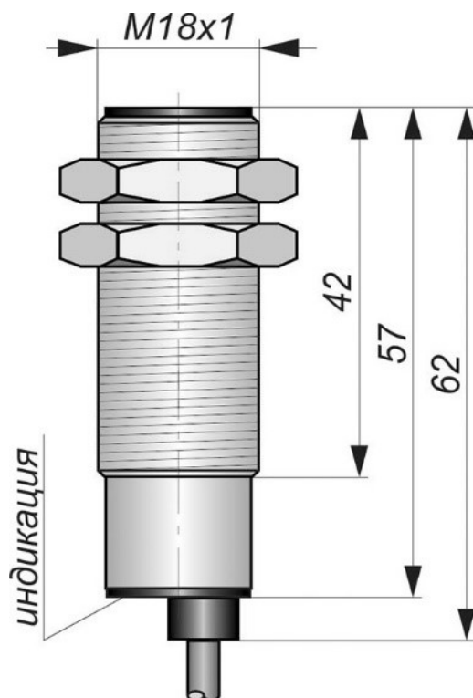
Габаритный чертеж
