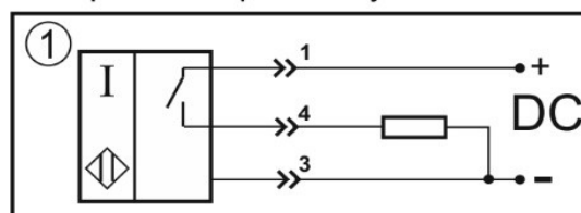
Нормально-разомкнутый контакт
