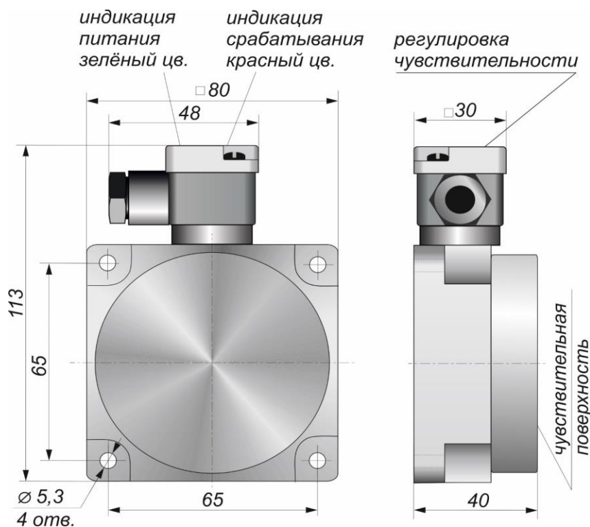
Габаритный чертеж
