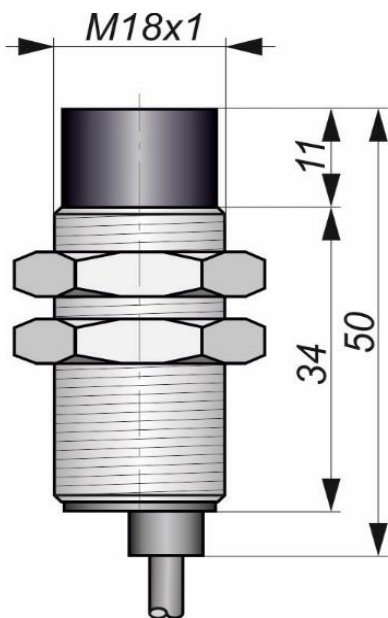
Габаритный чертеж
