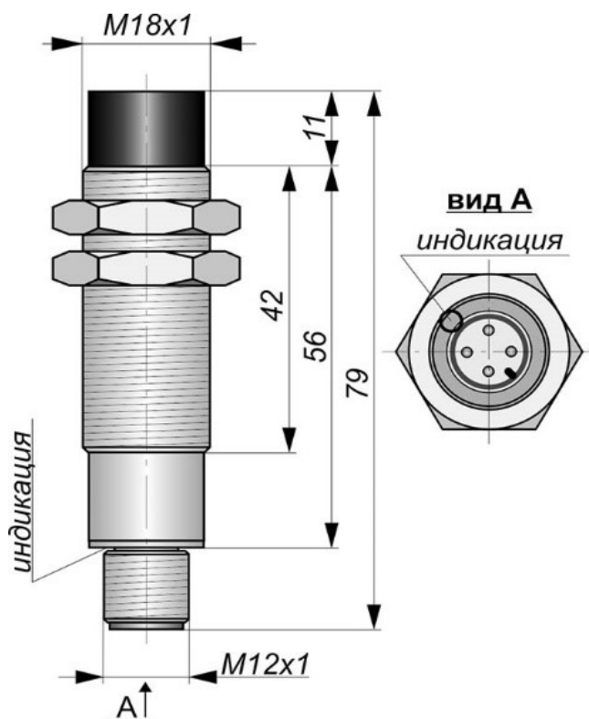
Габаритный чертеж
