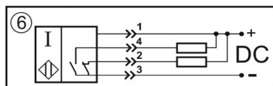
Переключающий контакт
