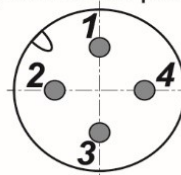
Цоколевка разъема
