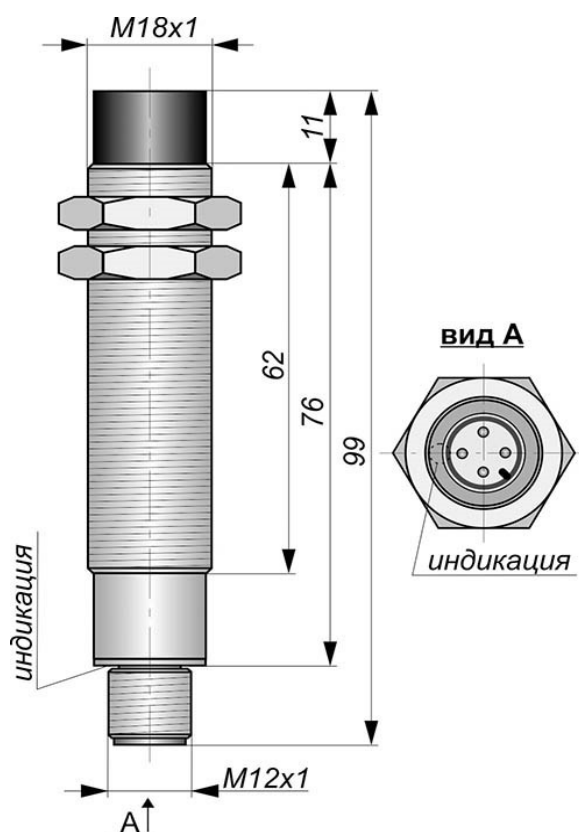
Габаритный чертеж
