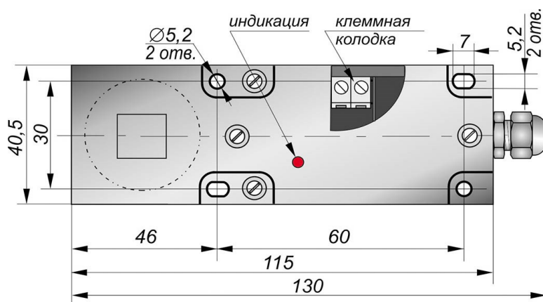
Габаритный чертеж
