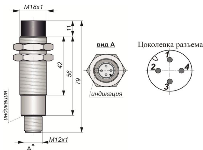
Габаритный чертеж
