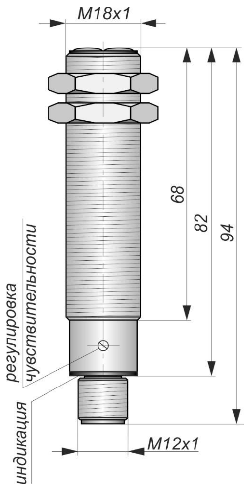
Габаритный чертеж
