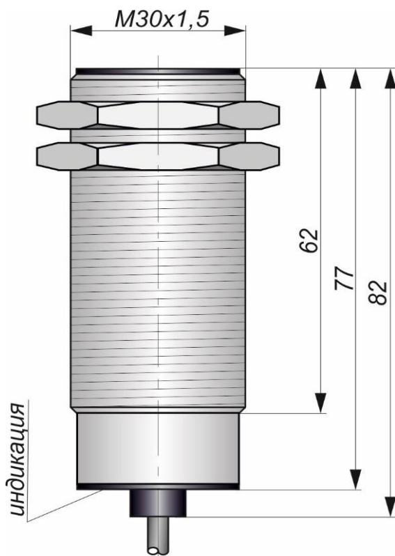
Габаритный чертеж
