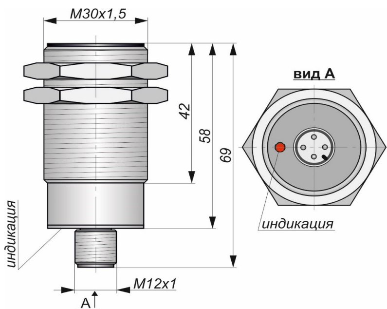
Габаритный чертеж
