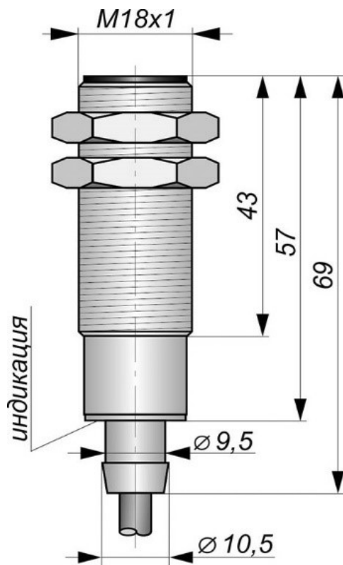
Габаритный чертеж
