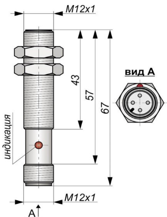
Габаритный чертеж
