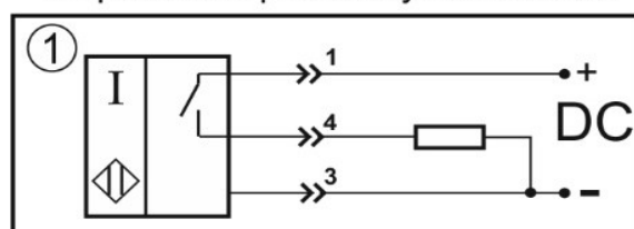
Цоколевка разъема
