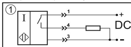
Цоколевка разъема
