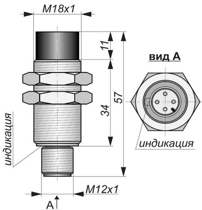
Габаритный чертеж
